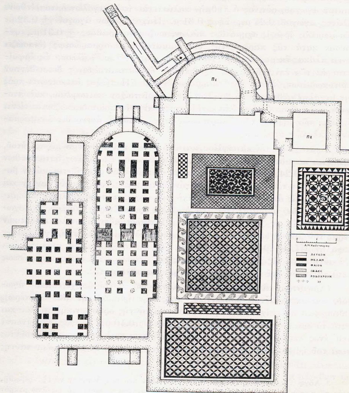
Εἰκ. 1. Κάτοψις τοῦ ρωμαϊκοῦ λουτροῦνος παρὰ τὸ Νησι Ἀλεξανδρείας.
